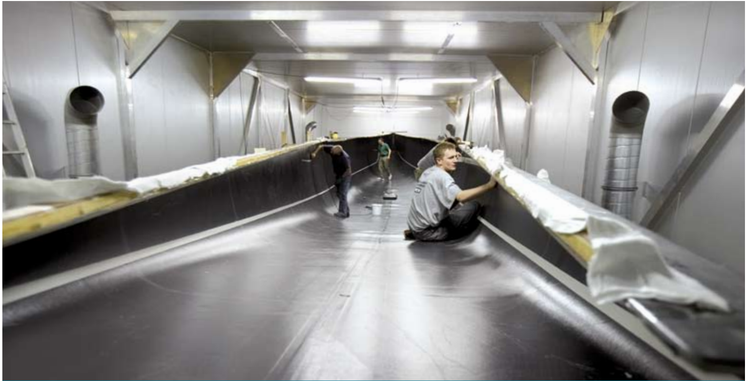
Der Aufbau unserer Rumpfschalen: Karbon-Innenlage, Sandwich-Material und Karbon-Außenlage.
